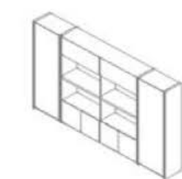
文件柜 EY98.3200 Cabinet W3200*D400*H1950
