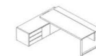
经理桌 EY86 Manager Table W2200*D1800*H750
