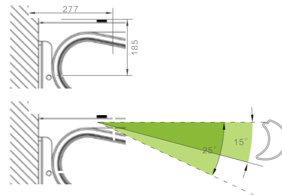
建议 (Proposal) : 15°~25°
