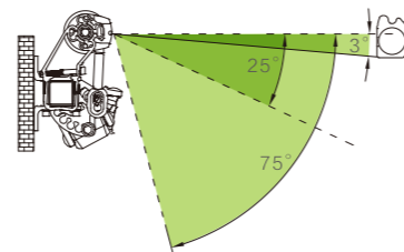
建议 ( Proposal ) : 15°~25°
