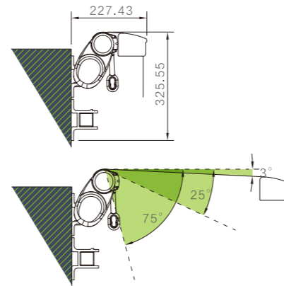
建议 ( Proposal ) : 15°~25°
