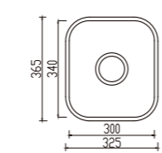
YH262A unit:mm
