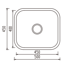
YH216A unit:mm
