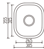
YH209A unit:mm
