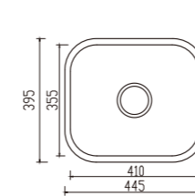
YH215A unit:mm
