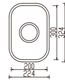
YH207A unit:mm
