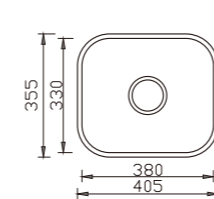
YH238A-2 unit:mm
