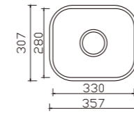
YH212A unit:mm
