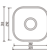
YH243A unit:mm
