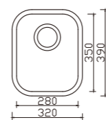
YH211A unit:mm
