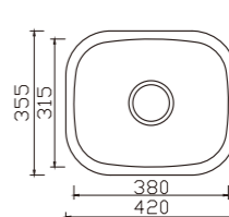
YH245A-2 unit:mm
