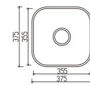
YH213A unit:mm
