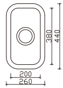
YH206A unit:mm
