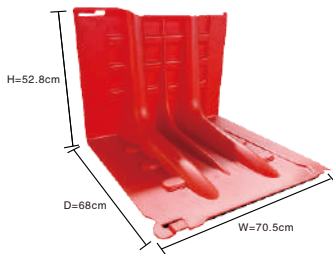
DW-WZ50直板挡水板
