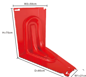
DW-NW75内弯挡水板
