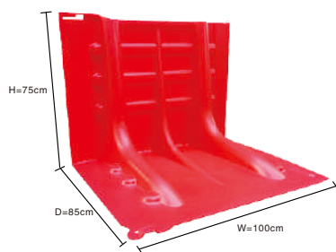
DW-WZ75直板挡水板
