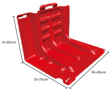
DW-WZ60直板挡水板
