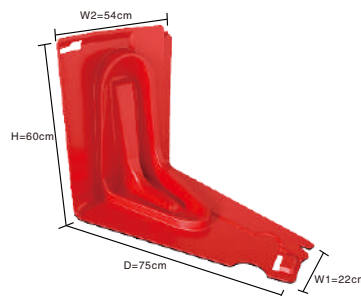
DW-NW60内弯挡水板
