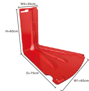
DW-WW60外弯挡水板
