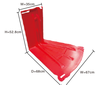
DW-WW50外弯挡水板
